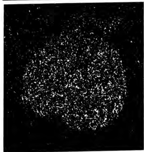
As.K \alpha
