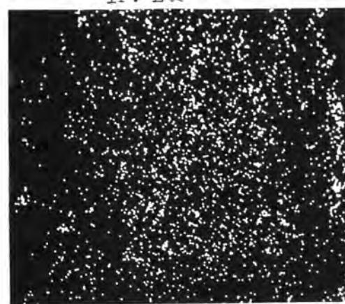
Ru.Lα
