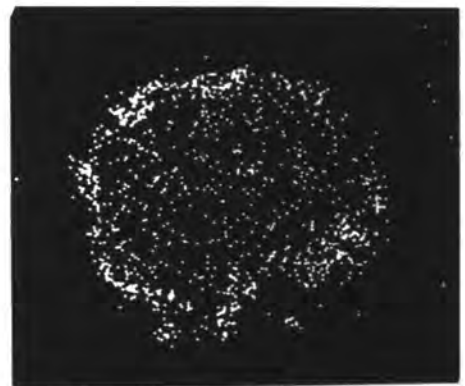
Ru.L \alpha
