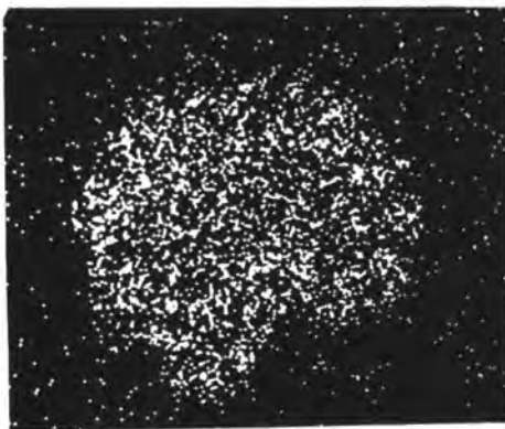
As.K \alpha
