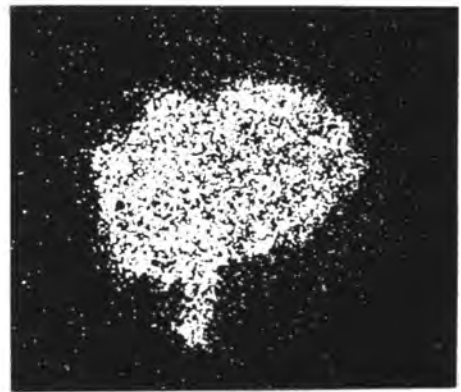
Ir.L \alpha
