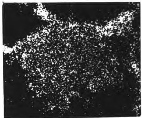
S.K \alpha
