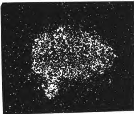
Pt.L \alpha
