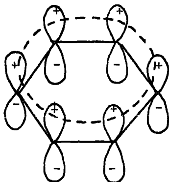
Hückel
