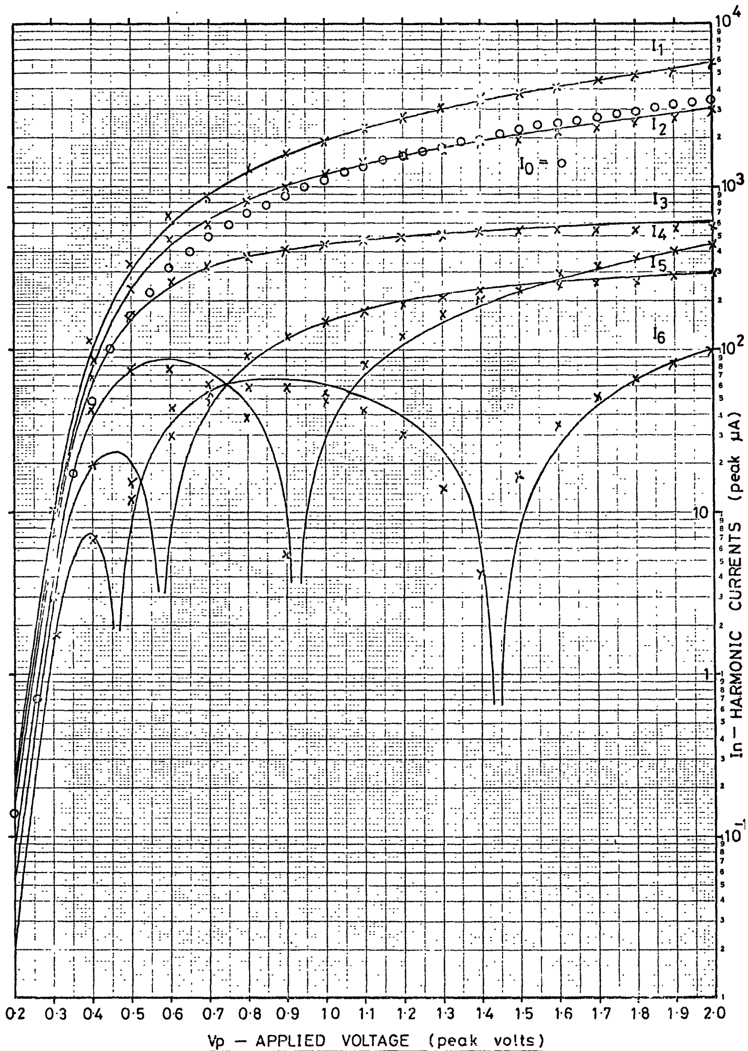
FIG. 6.17 DIODE TYPE 5082 - 2833 - C1
