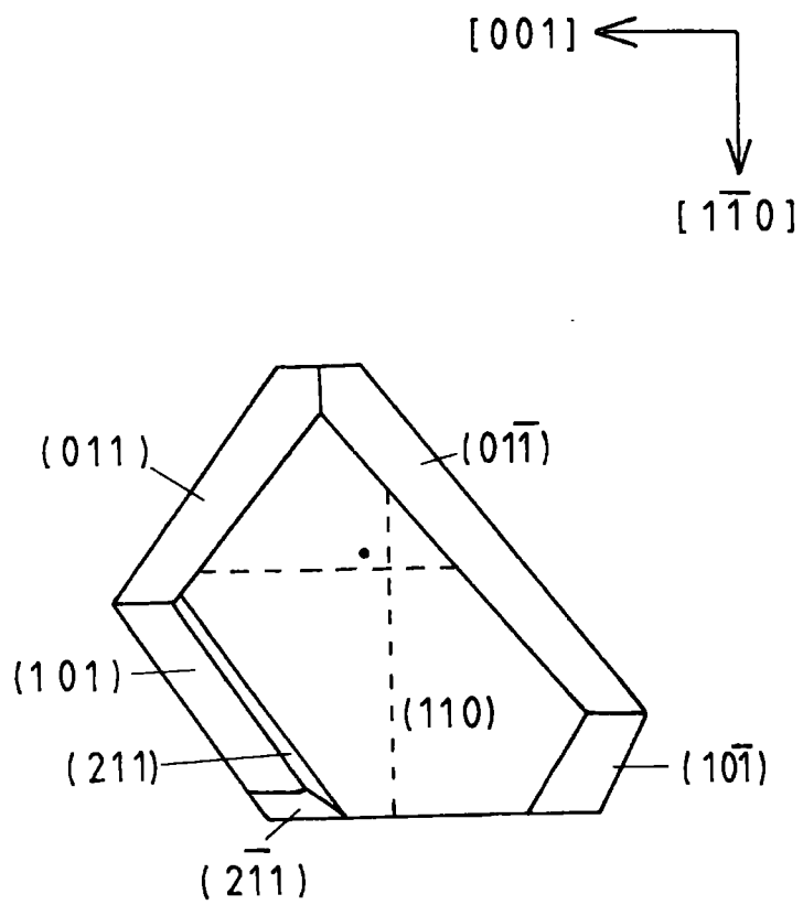
Fig. 5.3 Garnet Crystal
