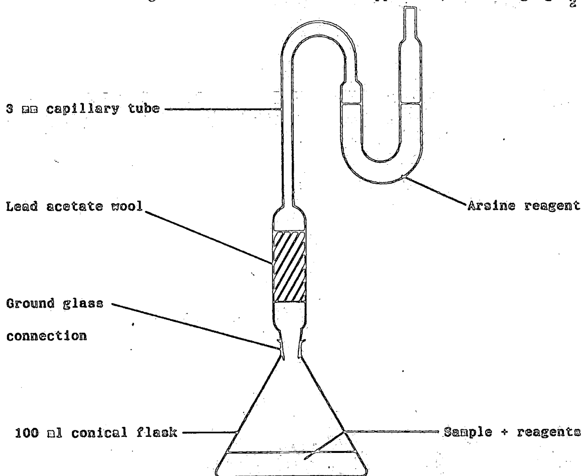
Fig. 3.561. The wet oxidation apparatus.
