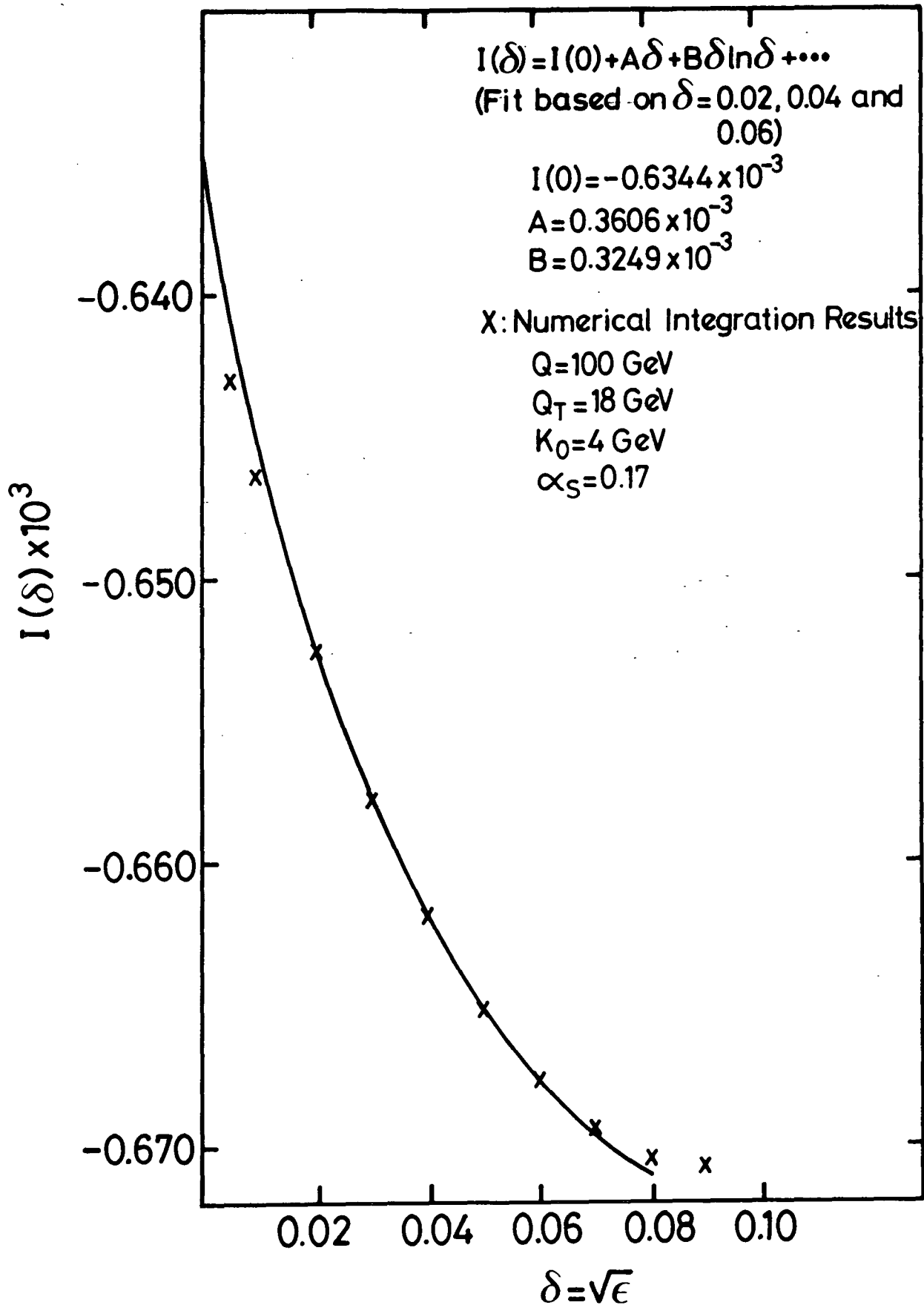
Figure V.2.3 : \epsilon -extrapolation
