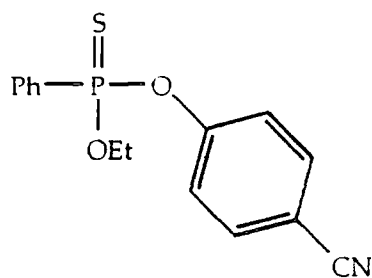
Cyanofenfos
