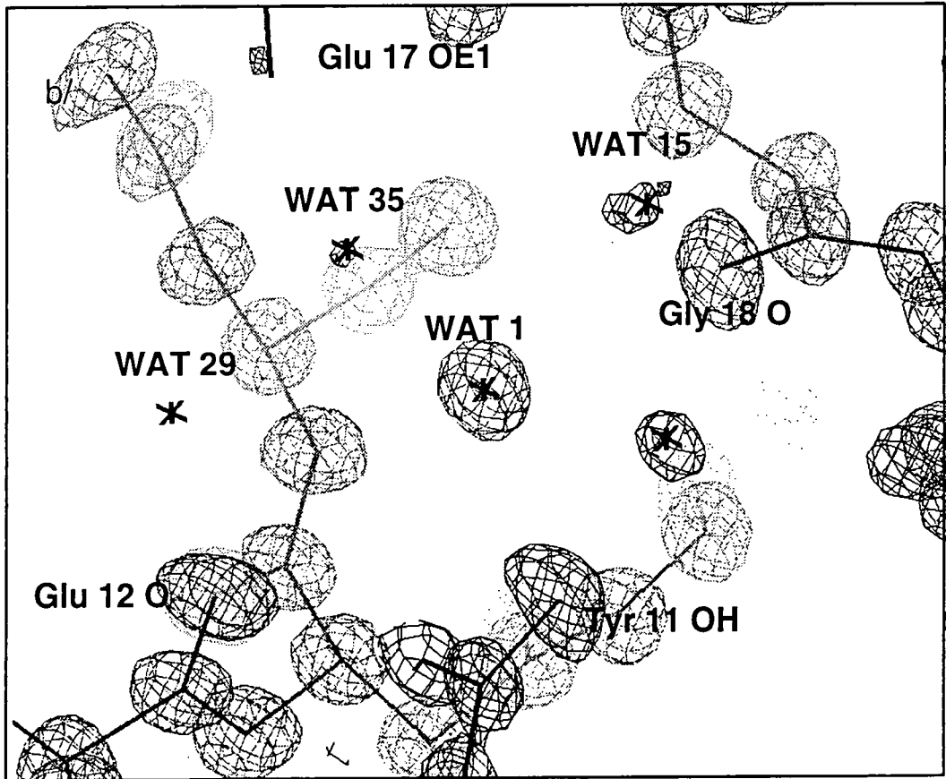
Figure 9. rubredoxin: a/ 3Fo - 2Fc b/ 3Eo - 2Ec map
