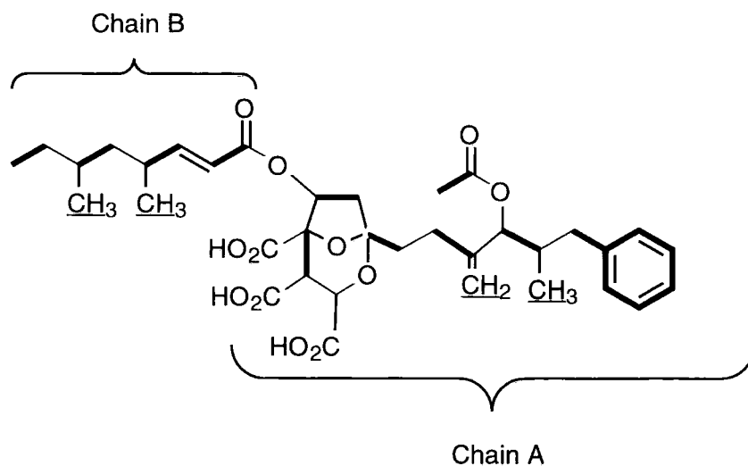
Scheme 1.4.1
