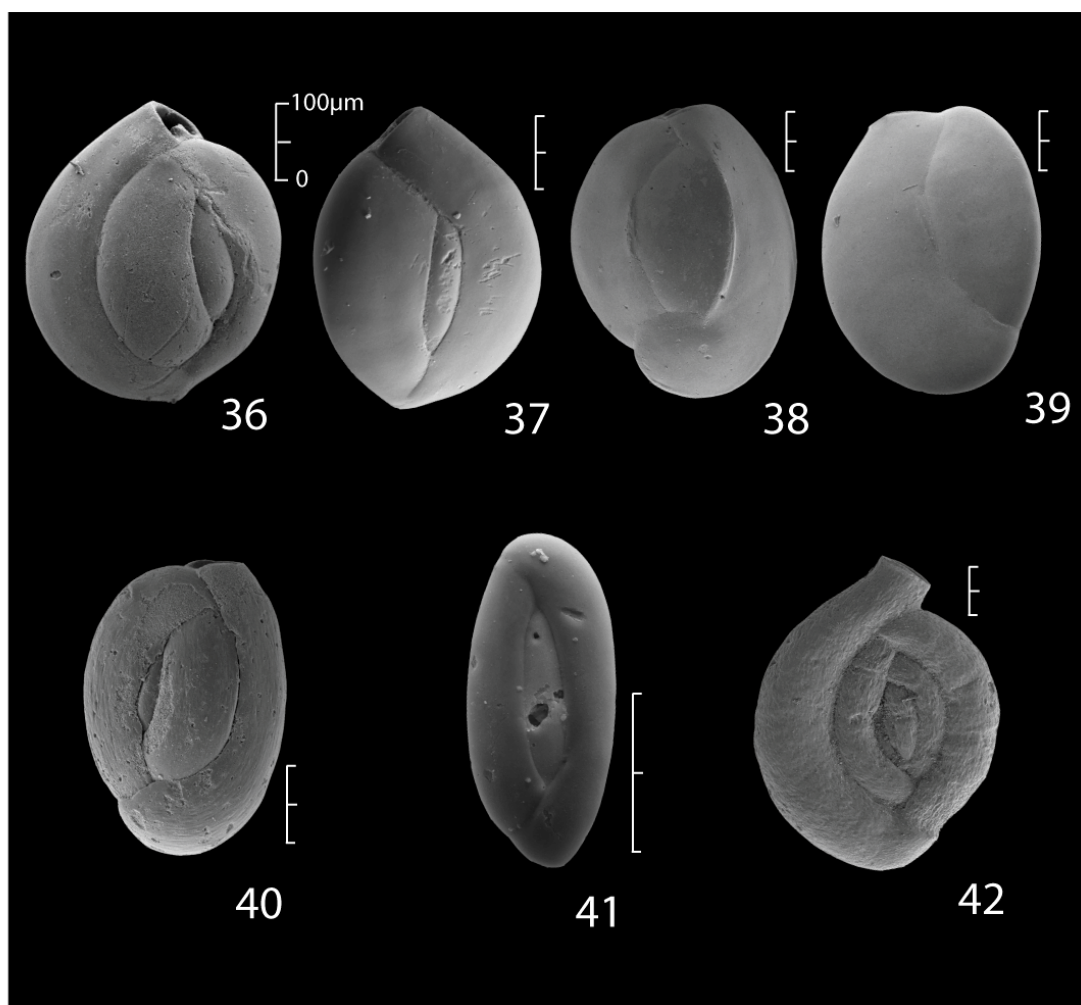
36, 37. Quinqueloculina akneriana d'Orbigny, 1846; 38, 39. Quinqueloculina lamarckiana d'Orbigny, 1839; 40. Quinqueloculina seminula Linné, 1758; 41. Quinqueloculina elongata Natland, 1938; 42. Spiroloculina lucida Cushman and Todd, 1944
