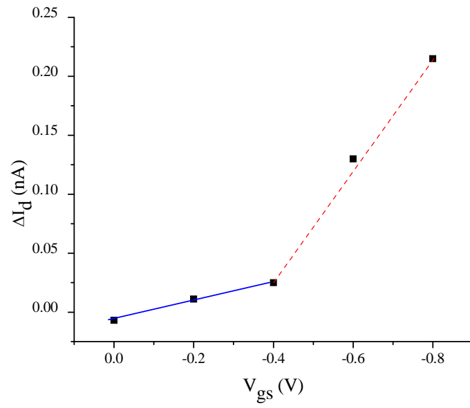
Figure 5.12 \Delta I_d versus V_{gs} , V_{ds} = 0 V, the standard ISOFET, in DI water.
