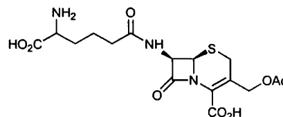
5 Cephalosporin C
