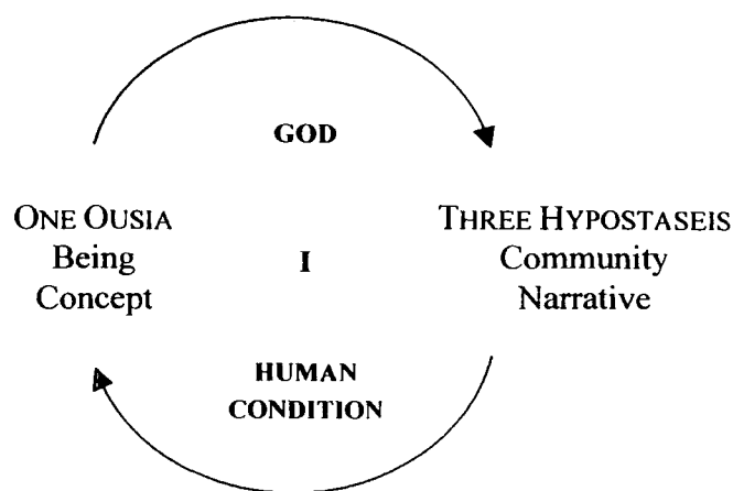
Graph 12: Trinitarian Gestaltkreis
