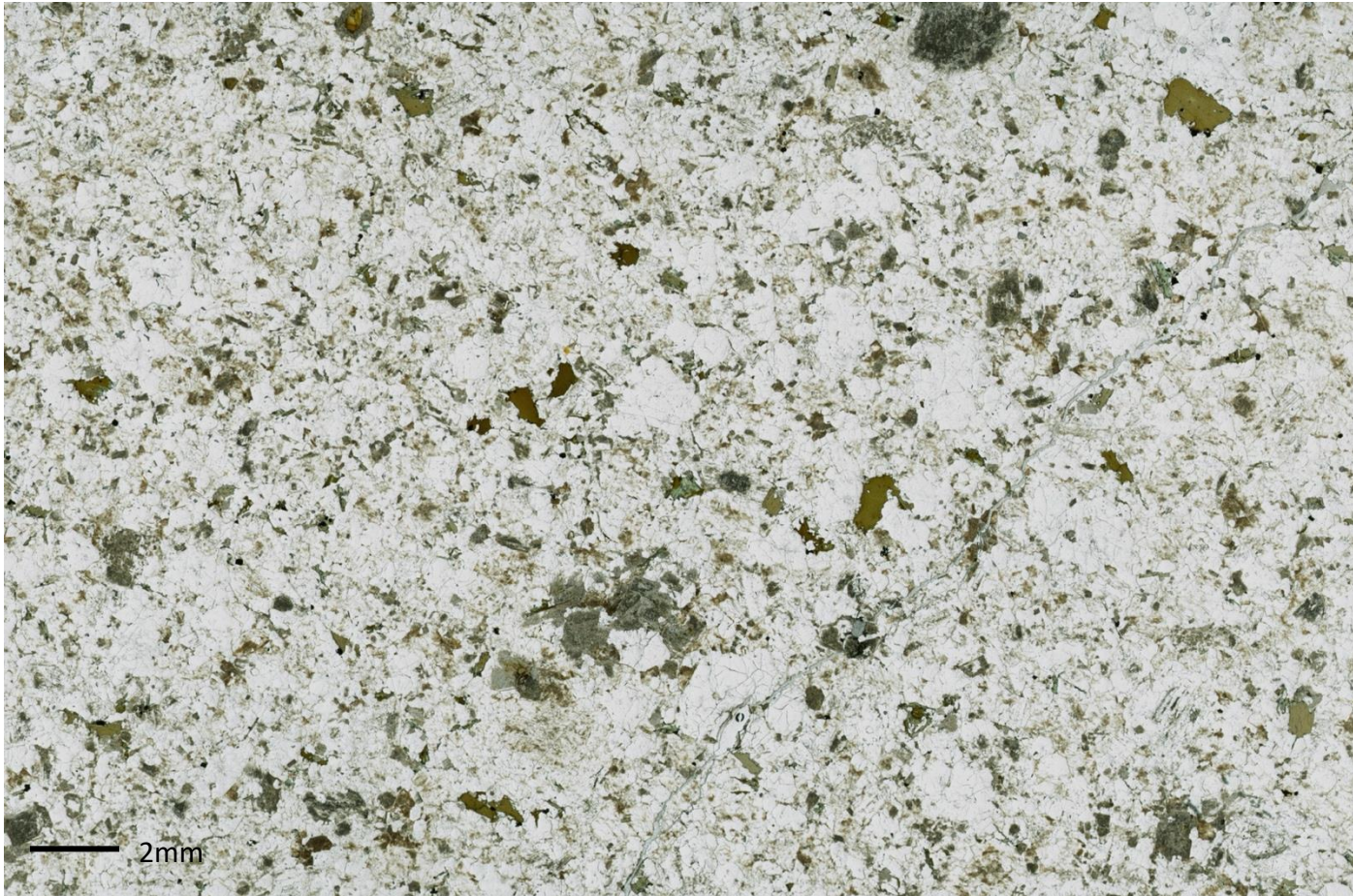
BP42 - Aplite
