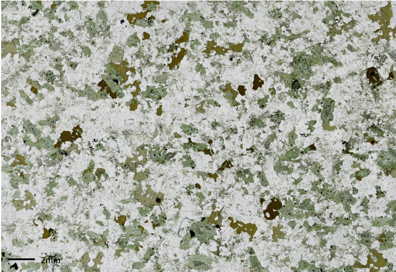
BP23 - Granodiorite
