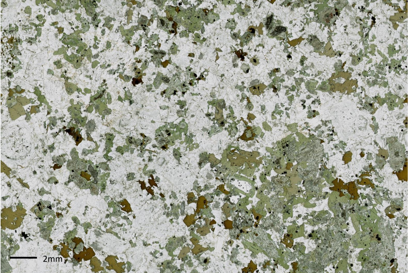
BP40 - Granodiorite
