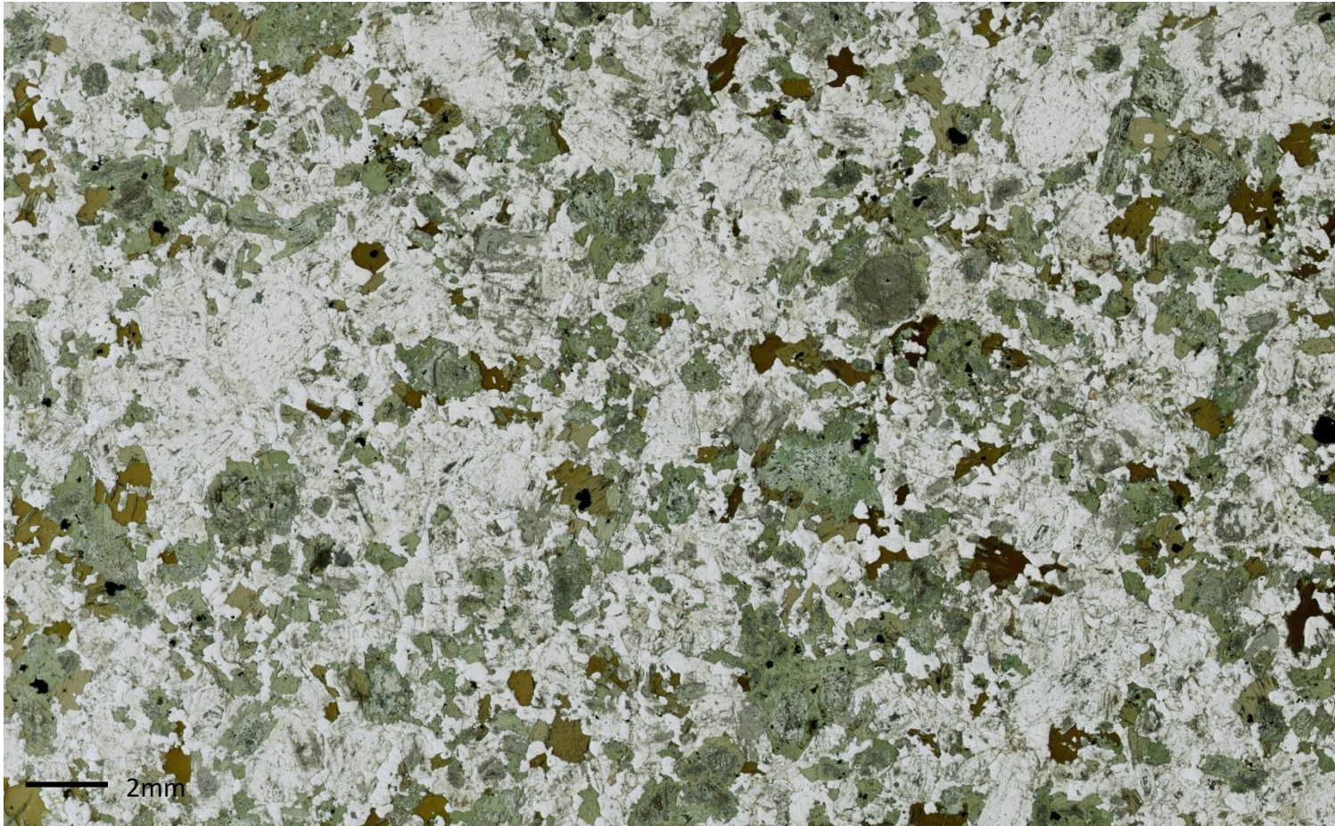
BP26 - Granodiorite
